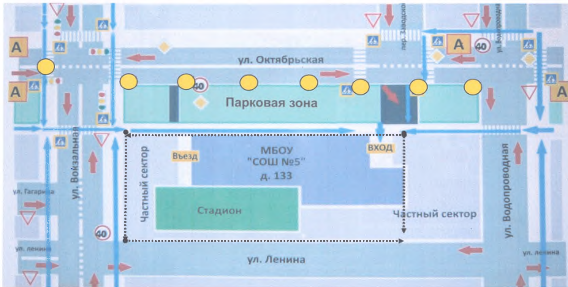
Схема организации дорожного движения в непосредственной близости от образовательной организации с размещением соответствующих технических средств организации дорожного движения, маршрутов движения детей и расположения парковочных мест
